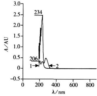
图 2 \text{ReO}_4^- 的紫外-可见光谱
