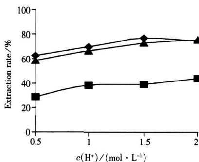
图1 不同酸体系及 \text{H}^+ 浓度对萃取率的影响
