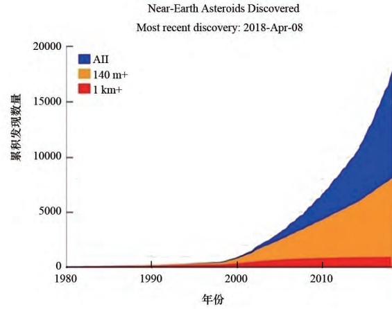
图2 近地小行星的直径、数量和发现时间的统计
