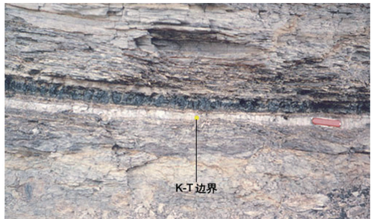
图6 西藏拉萨岗巴地区白垩系和第三系的界面层
