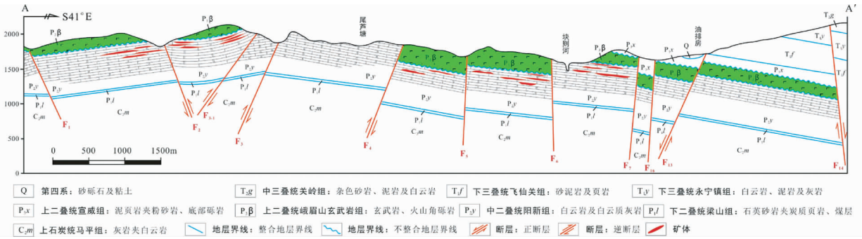
图 3 富乐铅锌矿集区 A-A' 剖面图 (据 Zhou et al. , 2018)
