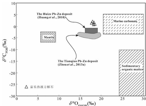
图6 富乐铅锌矿床 \delta^{13}\text{C}_{\text{PDB}}-\delta^{18}\text{O}_{\text{SMOW}} 图解 (转引自 Zhou et al. , 2013a)
