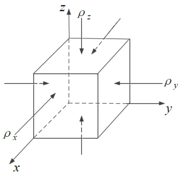
图 1 煤样三方向电阻率示意图
