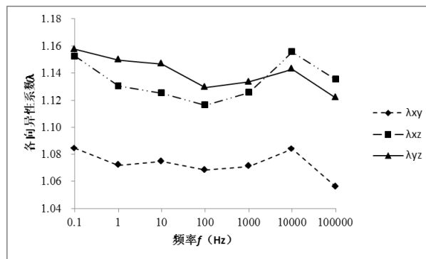
图 3 不同频率下的各向异性系数
