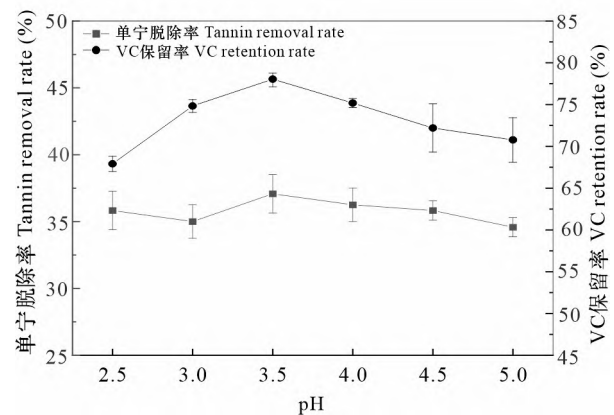
图 2 pH 值对单宁脱除率和 VC 保留率的影响 Fig. 2 Effects of pH on tannin removal rate and VC retention rate
