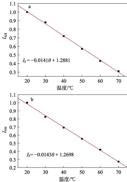
SP 溶液浓度为 1 μmol/L, λ ex = 360(OP)、750(TP) nm 图 7 SP 在 OPE (a) 和 TPE (b) 中的荧光强度对温度的线性拟合线 Fig. 7 Linear fitting lines of fluorescence intensity of SP to temperature in OPE (a) and TPE (b)
