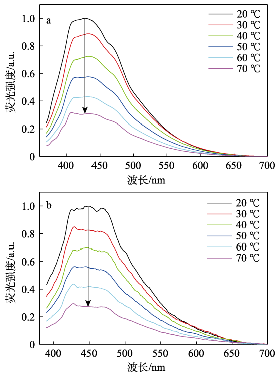
SP 溶液浓度为 1 μmol/L, λ ex = 360(OP)、750(TP) nm 图 6 SP 甘油溶液在 OPE (a) 和 TPE (b) 中的荧光强度与温度的关系 Fig. 6 SP in glycerol OPE (a) and TPE (b) fluorescence intensity in relation to temperature
