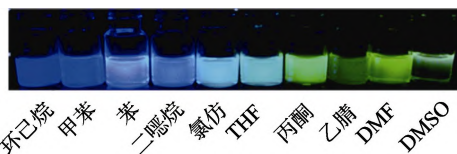
图 3 SP 在不同溶剂中的荧光照片 ( c = 10 \mu\text{mol/L} , \lambda_{\text{ex}} = 365 \text{ nm} )
