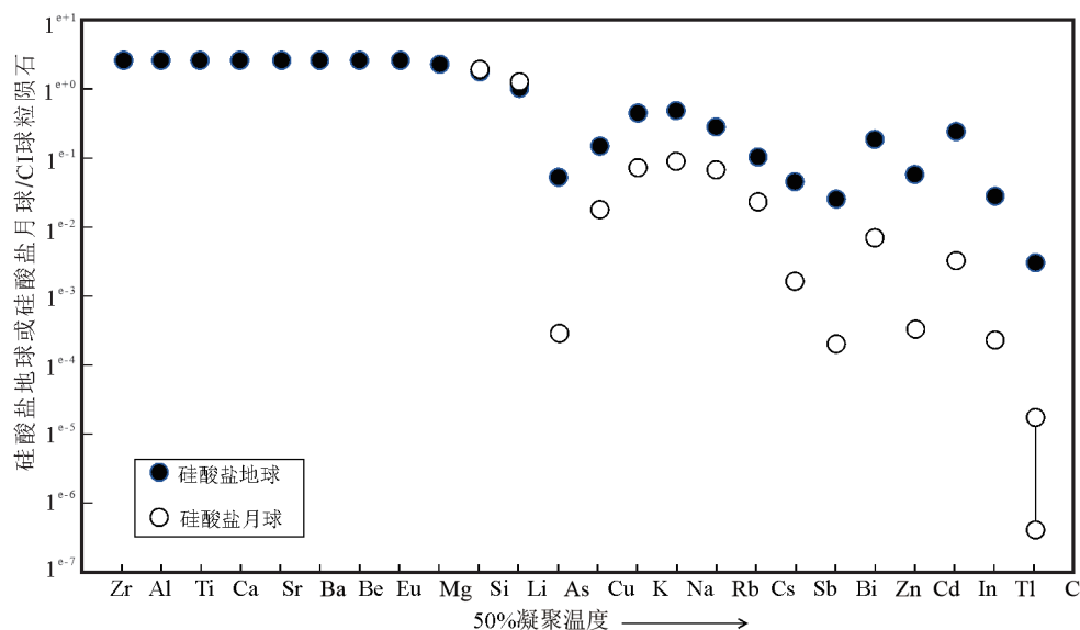
数据来源: 地球数据来自Palme和O'Neill(2014); 月球数据来自Taylor(1982), Taylor和Wieczorek(2014), Richter等(2011, 2018)
