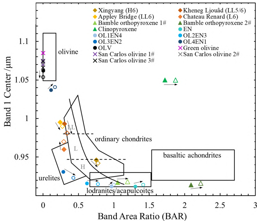
图2 1\ \mu\text{m} 吸收中心与吸收面积比.实心点为辐照前数据,空心点为辐照后数据(多次辐照的样品取累计能量最高的数据),箭头方向为模拟太空风化的效果趋势方向.
