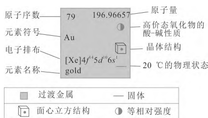
图1 Au元素的性质(修改自Encyclopaedia Britannica)
