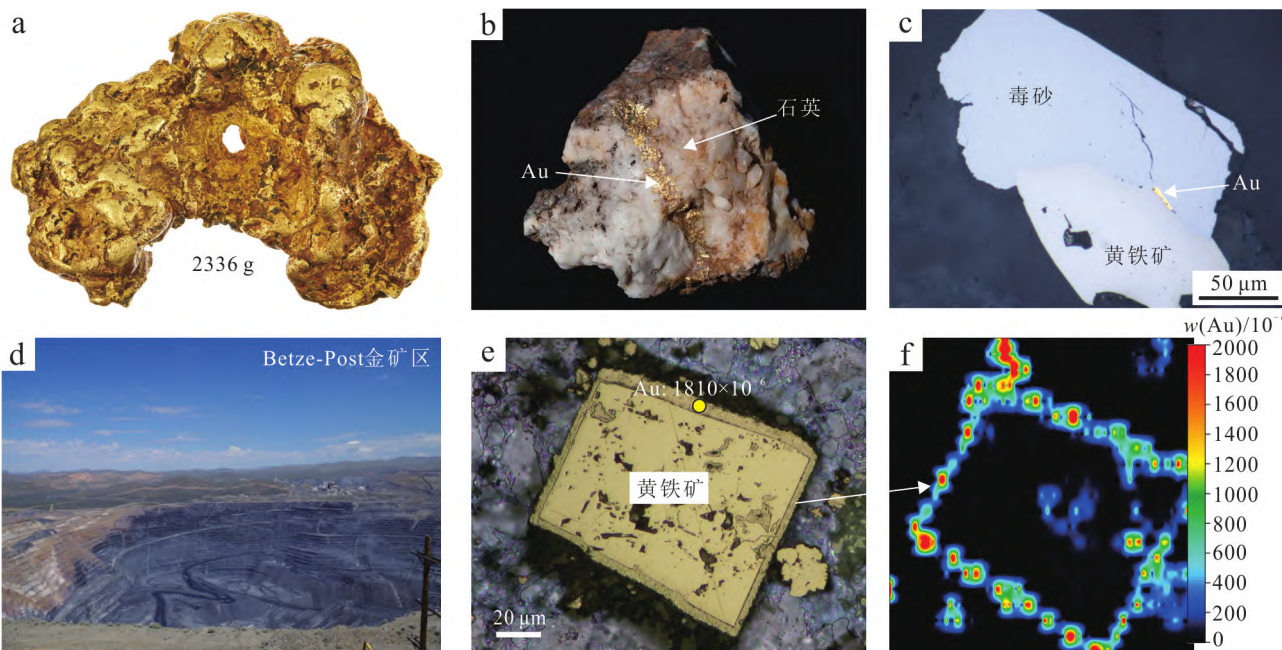
图 4 狗头金(a, 图片来源网络)、矿石手标本上显示出 Au 和石英共生(b, 图片来源网络)、光学显微镜下显示出 Au 和硫化物共生(c)、世界上储量最大的卡林型金矿采坑(d, 美国内华达州 Betze-Post 金矿, Au 储量: 1250 t)、卡林型金矿中的载金黄铁矿(e, Au 含量为电子探针分析所测得; Xie et al., 2018)和 Au 元素分布图(f, Au 含量通过激光电感耦合等离子质谱仪获得; Xie et al., 2018)
