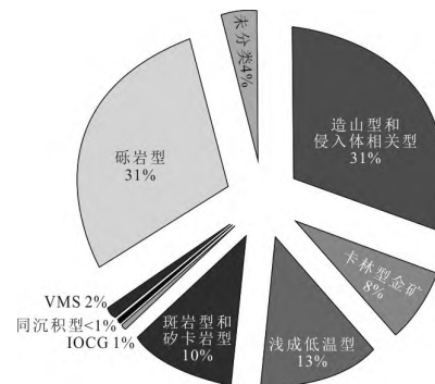
图 3 不同类型金矿的产出占比(修改自 Frimmel, 2008)
