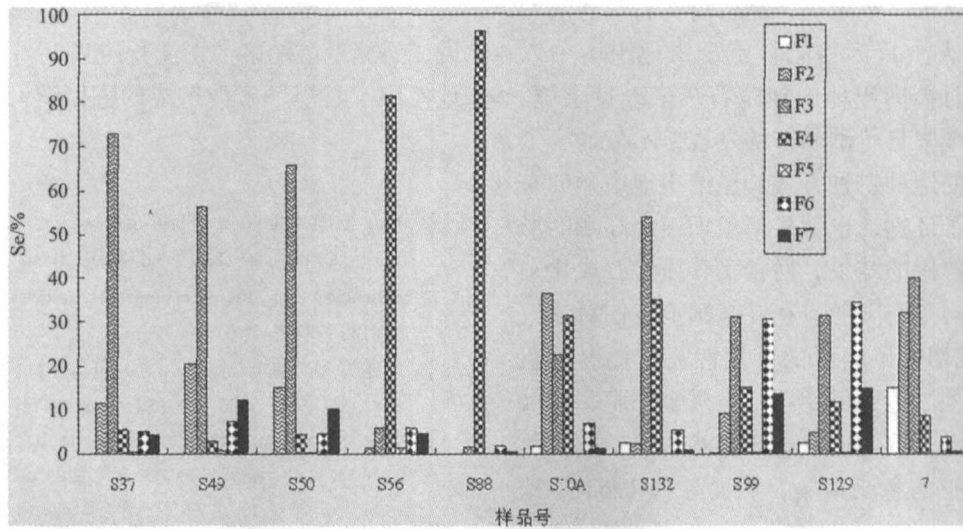
图1 渔塘坝土壤硒的结合态分布
