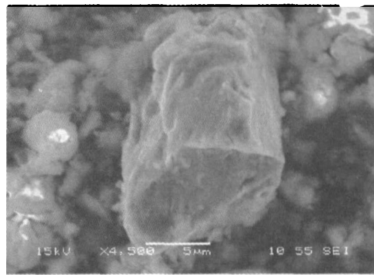
图2 S88土壤样品中的自然硒晶体(SEM-SEI照片)
