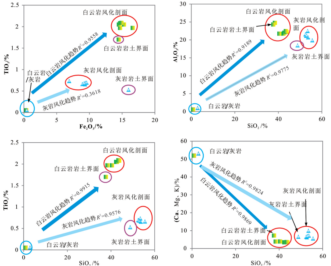
图7 白云岩剖面和灰岩剖面不同元素的质量含量散点图及风化趋势
