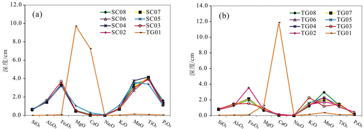
图4 白云岩和石灰岩剖面主要元素上地壳元素平均值(UCC)标准化蜘蛛图
