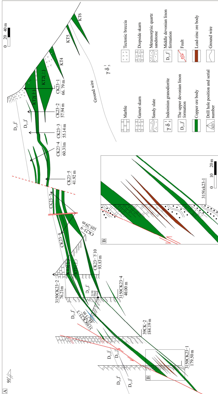
图 2 羊拉铜矿床里农矿段 23 号勘探线剖面图 [29]
