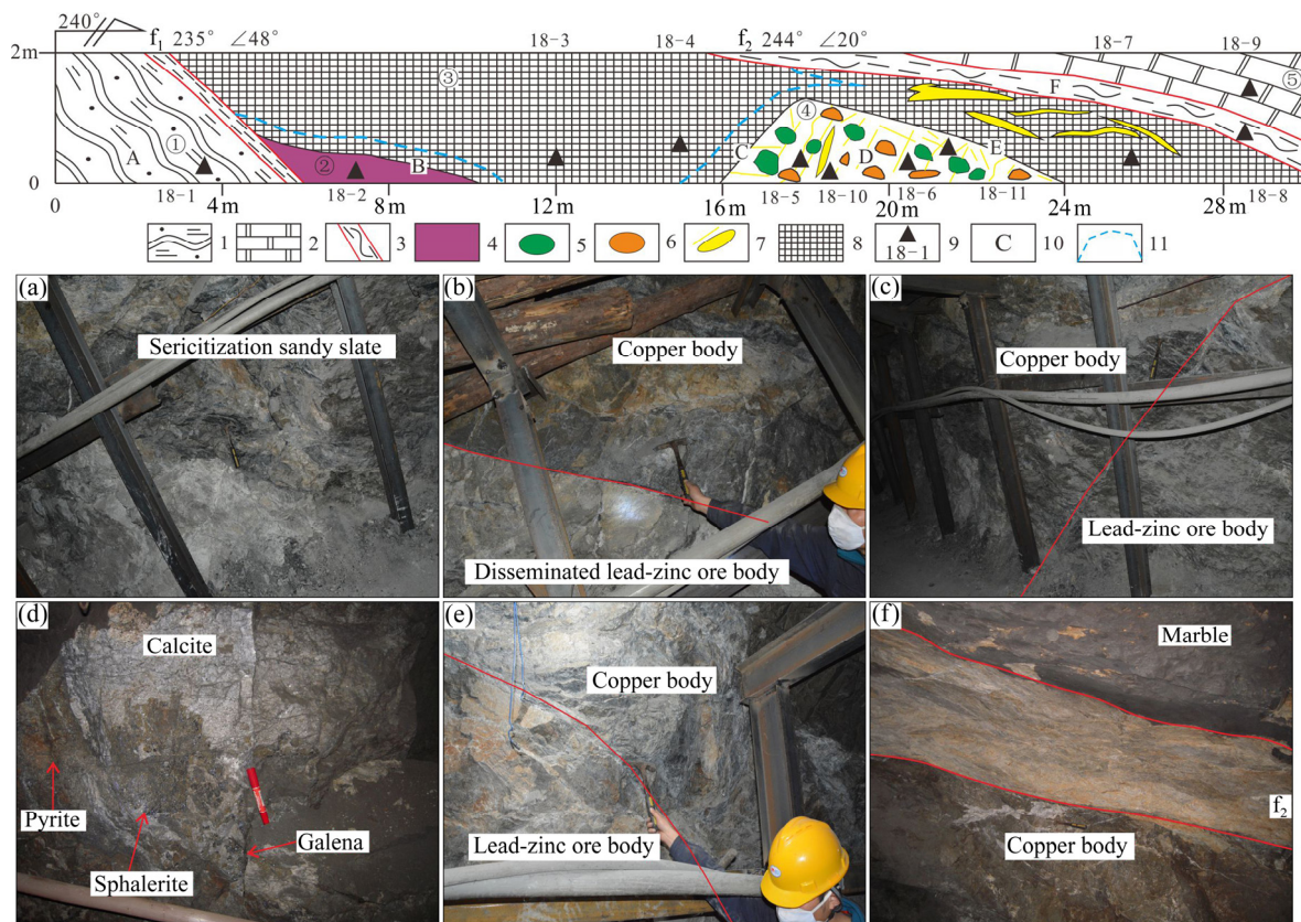
图 3 羊拉铜矿床 3100 m 中段 18#穿脉铅锌矿体素描图
