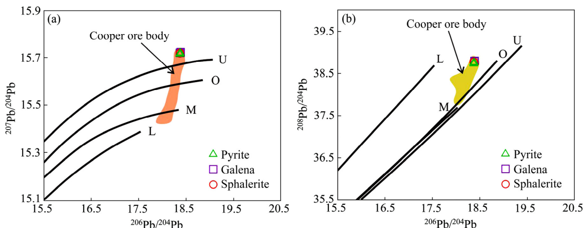
图 15 羊拉矿床矽卡岩铅锌矿体和矽卡岩铜矿体的 ^{207}\text{Pb}/^{204}\text{Pb}-^{206}\text{Pb}/^{204}\text{Pb} 图(a)和 ^{208}\text{Pb}/^{204}\text{Pb}-^{206}\text{Pb}/^{204}\text{Pb} 图(b) (图中数据来源见表 7, 底图据文献[88]): U—上地壳; O—造山带; M—地幔; L—下地壳
