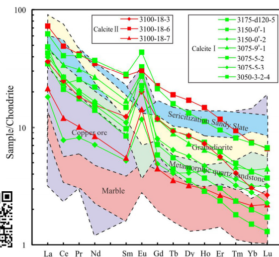
图 9 羊拉铜矿床铜矿石、大理岩、绢云砂质板岩、变质石英砂岩、花岗闪长岩及铅锌矿石中方解石稀土元素配分图(球粒陨石标准值据文献[37])
