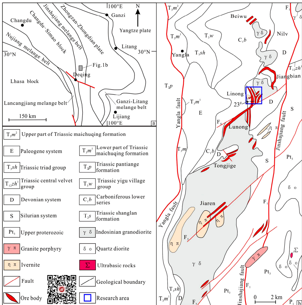
图1 羊拉铜矿床大地构造位置和矿区地质简图 [1]
