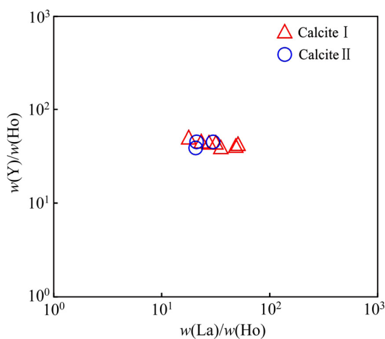
图 8 羊拉铜矿铅锌矿石中方解石的 w(Y)/w(Ho)-w(La)/w(Ho) 关系图 [55]
