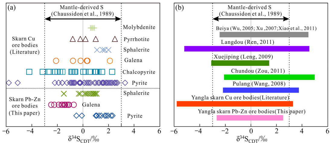
图 12 羊拉铜矿床矽卡岩型铅锌、铜矿体的 S 同位素组成(a)以及幔源 S 和三江成矿带典型矿床的 S 同位素组成(b) [77-84]
