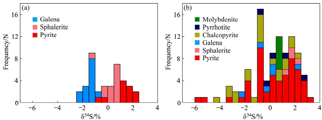
图 14 羊拉矿床矽卡岩型铅锌矿体 S 同位素直方图(a)和羊拉矿床矽卡岩型铜矿体 S 同位素直方图(b)
