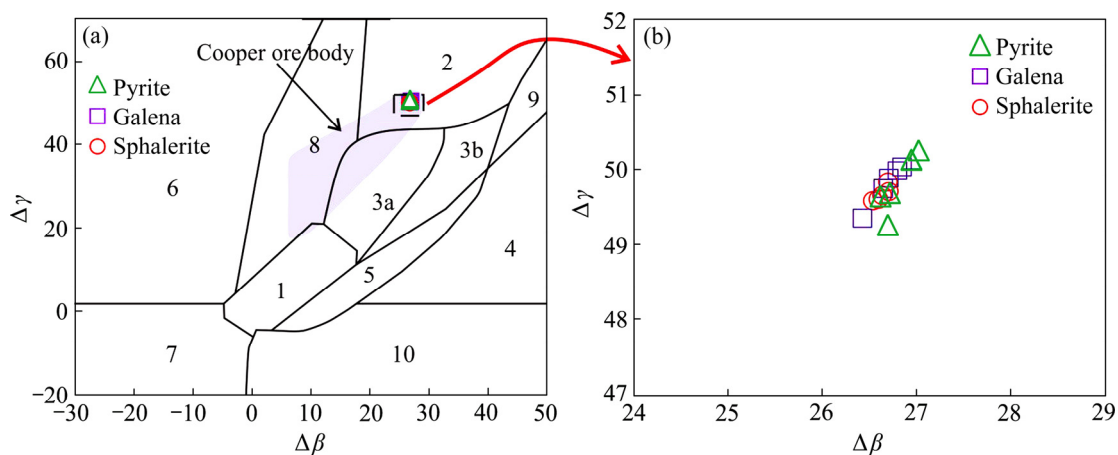
图 16 羊拉矿床矽卡岩型铅锌矿体和铜矿体的铅同位素 \Delta\gamma-\Delta\beta 图解(图中数据来源见表 7, 底图据文献 [87] ): (a) 矽卡岩型铅锌矿体和铜矿体; (b) 矽卡岩型铅锌矿体; 1—地幔源铅; 2—上地壳源铅; 3—上地壳与地幔混合的俯冲带铅(3a—岩浆作用; 3b—沉积作用); 4—化学沉积型铅; 5—海底热水作用铅; 6—中-深变质作用铅; 7—深变质下地壳铅; 8—造山带铅; 9—古老页岩上地壳铅; 10—退变质作用铅
