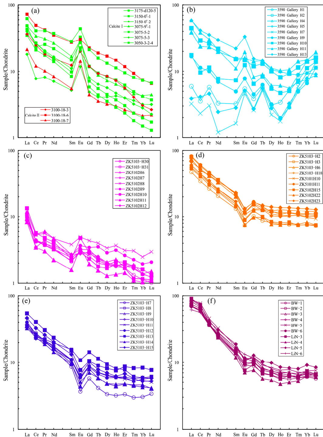
图6 羊拉铜矿床铜矿石、大理岩、绢云砂质板岩、变质石英砂岩、花岗闪长岩及铅锌矿石中方解石稀土元素配分图(球粒陨石标准值据文献[37]): (a) 方解石; (b) 铜矿石; (c) 大理岩; (d) 绢云砂质板岩; (e) 变质石英砂岩; (f) 花岗闪长岩
