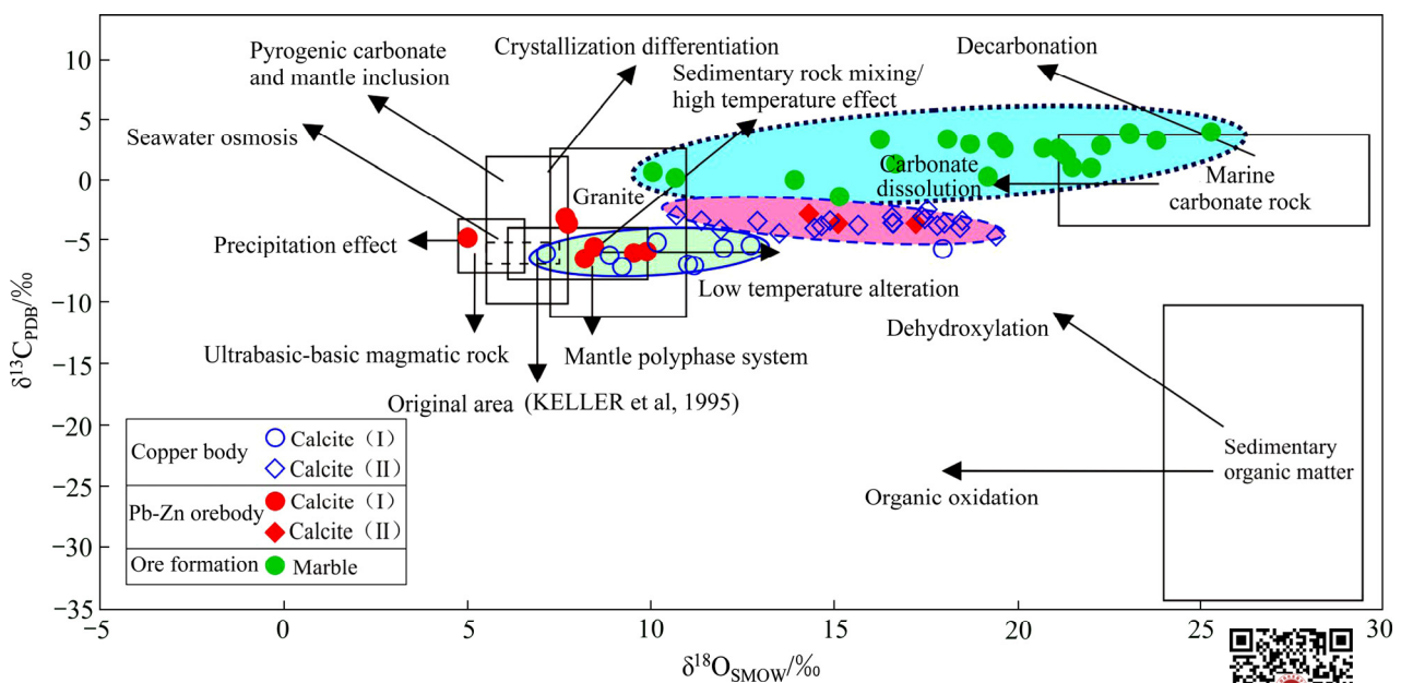
图 10 羊拉铜矿床铅锌矿石中方解石的 \delta^{18}O - \delta^{13}C 图(底图据文献[61])
