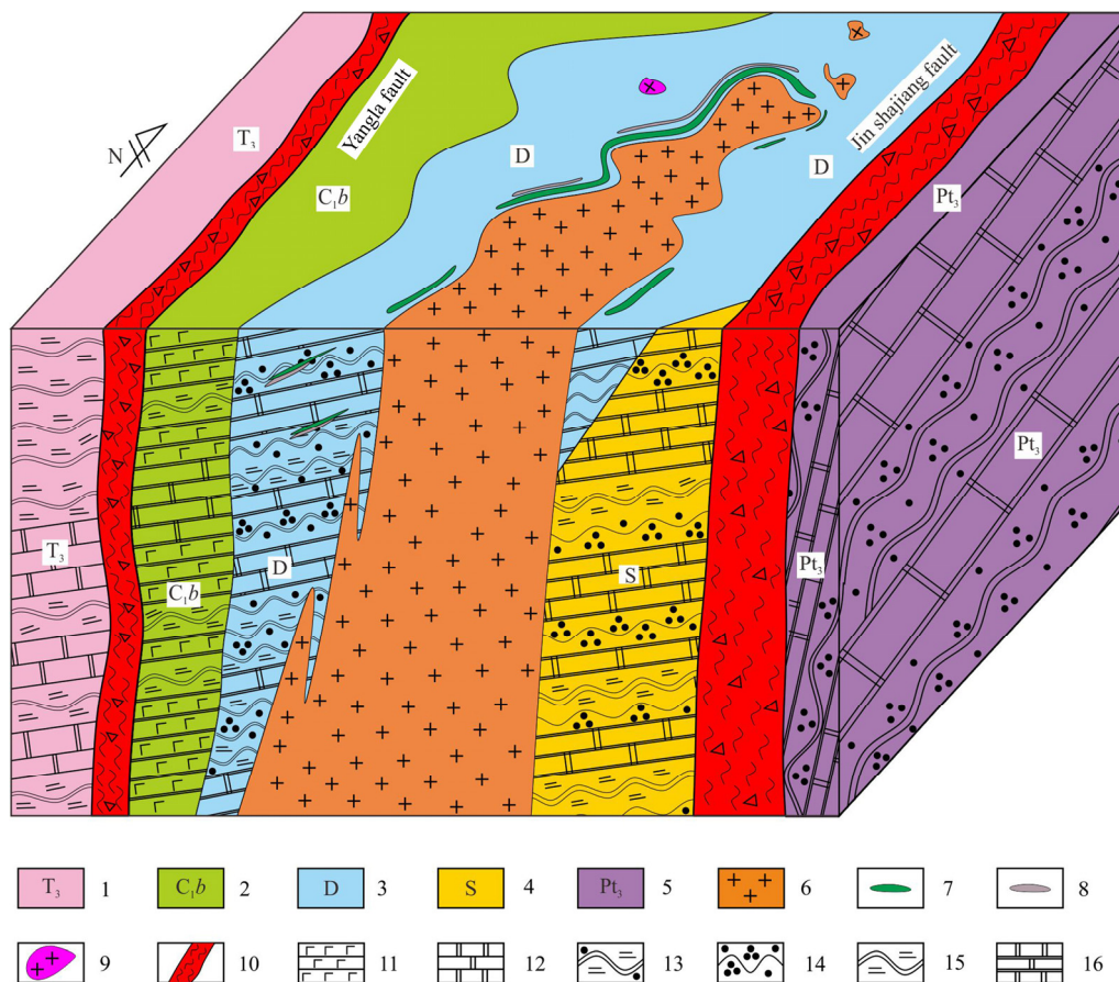
图 19 羊拉矿床铜铅锌成矿模式图: 1—三叠系; 2—石炭系贝吾组; 3—泥盆系; 4—志留系; 5—新元古界; 6—花岗闪长岩; 7—铜矿体; 8—铅锌矿体; 9—花岗斑岩; 10—断裂; 11—玄武岩; 12—灰岩; 13—绢云砂质板岩; 14—变质石英砂岩; 15—板岩; 16—大理岩
