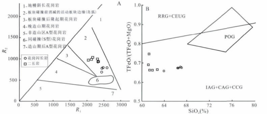
TFeO-全铁; IAG+CAG+CCG-岛弧花岗岩类+大陆弧花岗岩类+大陆碰撞花岗岩类; POG-后造山花岗岩; RRG+CEUG-裂谷花岗岩类+大陆造山后抬升阶段花岗岩类 图8 库喀阿孜铅-锌-(铜-钨)多金属矿区二长岩、花岗闪长岩的 R_1-R_2 图解(A) 和 TFeO/[(TFeO) + (MgO)] vs. SiO_2 图解(B)(据文献 [22,32] 修改)
