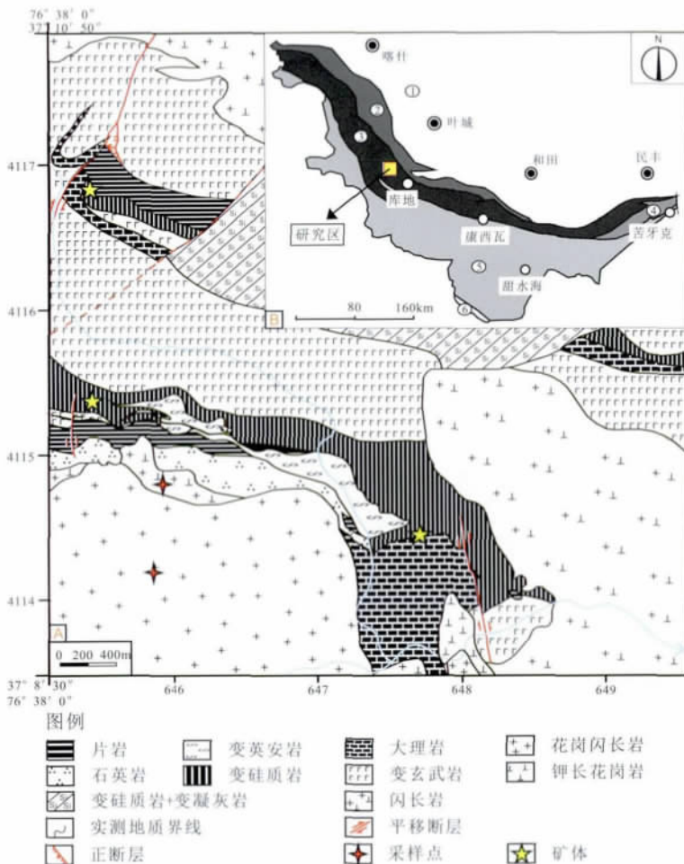
①-塔里木地块(华北板块); ②-北昆仑晚古生代陆缘裂谷带; ③-西昆仑中间地块及显生宙岩浆弧带; ④-上其汗早古生代岛弧带; ⑤-羌塘地块(华南板块); ⑥-冈底斯地块(印度板块)之空喀山口中生代陆缘盆地带
