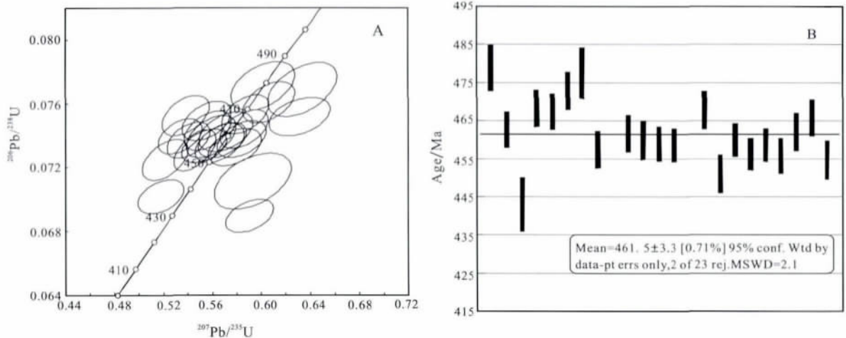
图7 库喀阿孜铅-锌-(铜-钨)多金属矿区二长岩的锆石 U-Pb 谐和年龄(A)和加权平均年龄(B)
