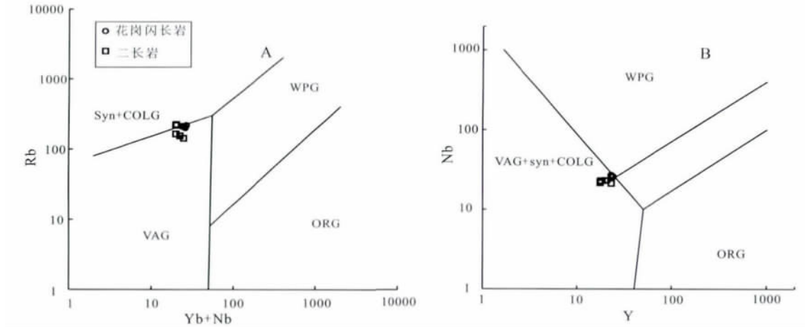
图9 库喀阿孜铅-锌-(铜-钨)多金属矿区二长岩、花岗闪长岩的 Rb-Yb+Nb 图解(A)和 Y-Nb 图解(B)(据文献[35]修改)
