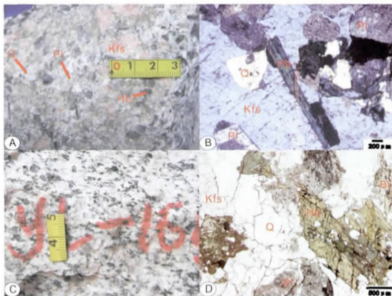
A-二长岩标本照片;B-二长岩的显微照片(正交偏光);C-花岗闪长岩标本照片;D-花岗闪长岩的显微照片(单偏光);Kfs-钾长石;Pl-斜长石;Hb-角闪石;Q-石英;Bi-黑云母
