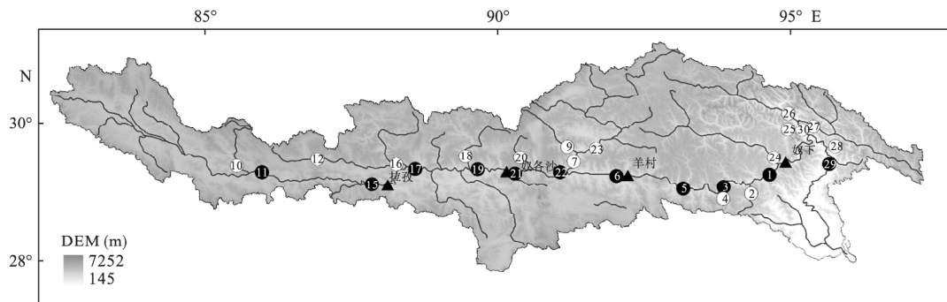
图1 雅鲁藏布江 CH 4 和 N 2 O 气体采样点示意图
