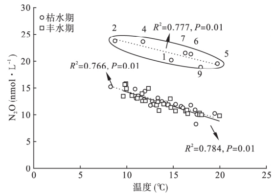
图 2 雅鲁藏布江中 N 2 O 浓度与水温的关系
