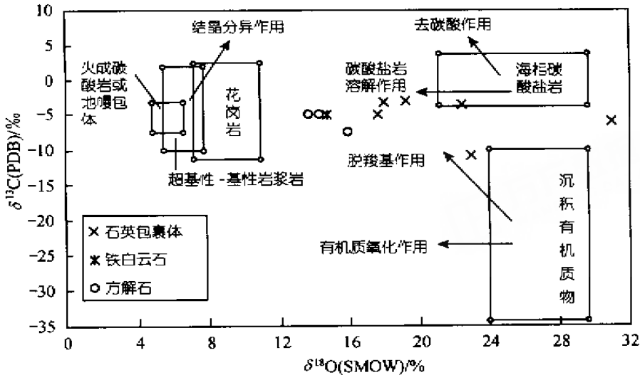
图 3 矿石中方解石、铁白云石以及石英流体包裹体的 \delta^{18}\text{O} - \delta^{13}\text{C} 图解
