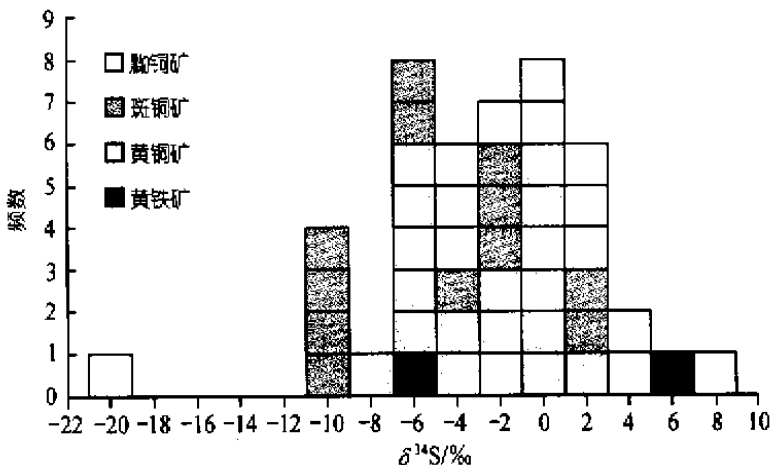
图 2 金满铜矿床硫同位素组成分布图
