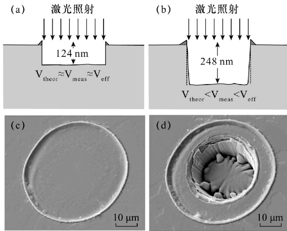
(a) 和 (b) 据文献 [75]; (c) 和 (d) 据文献 [33]。
