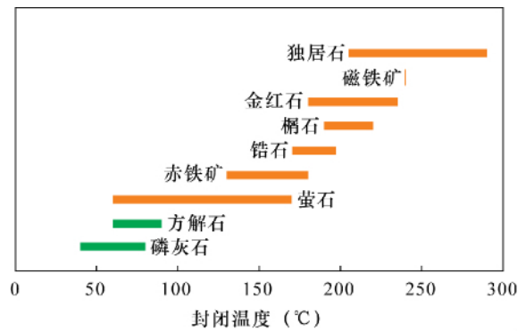
各矿物数据来源文献: 磷灰石 [77] ; 锆石 [78] ; 萤石 [20, 60, 79] ; 榍石 [54] ; 金红石 [63, 80-82] ; 独居石 [59, 83] ; 方解石 [61] ; 赤铁矿 [66] ; 磁铁矿 [4] 。
