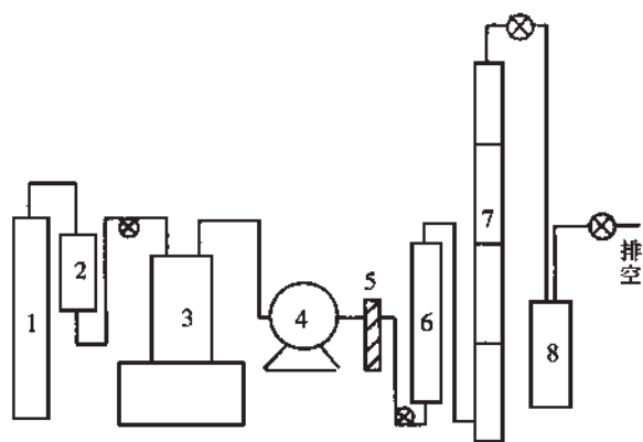
图 1 超临界 CO 2 萃取-精馏装置示意
