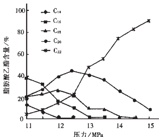
图 2 鱼油脂肪酸乙酯馏分与压力关系图
