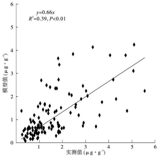
图 5 万山汞矿区居民头发甲基汞含量实测值和模型值之间的关系
