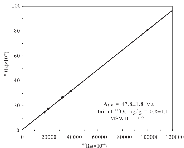
图5 连城Cu-Mo矿床Re-Os等时线图
