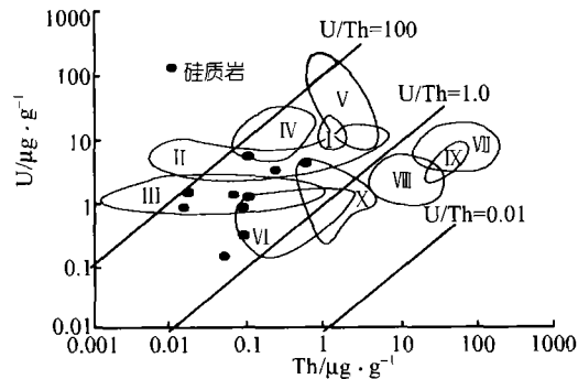
图 5 沉积物 U-Th 图解 [5,11]
