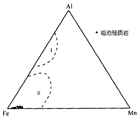
图 4 硅质岩成因的 Al-Fe-Mn 判别图解 [1,11]
