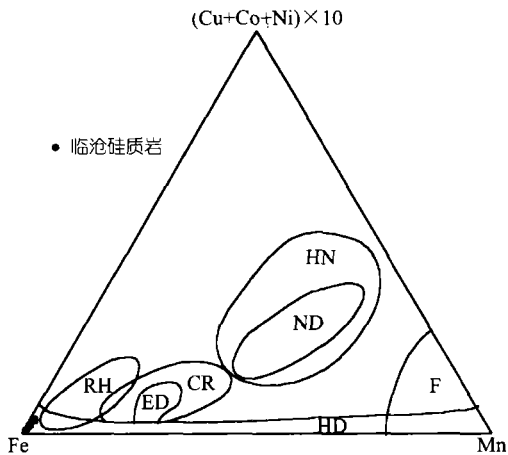
图 6 沉积物的 Fe-Mn-(Cu+Co+Ni) × 10 三角图解 [4]
