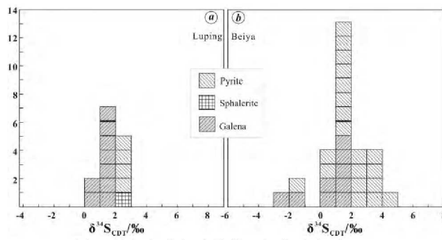
图2 炉坪与北衙硫化物 S 同位素组成
