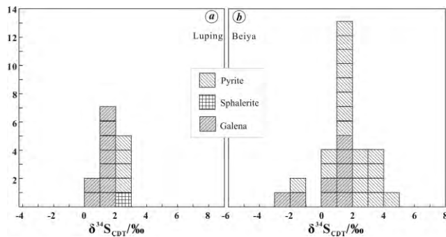
图 2 炉坪与北衙硫化物 S 同位素组成
