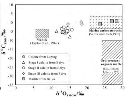
图 3 炉坪与北衙 C-O 同位素组成
