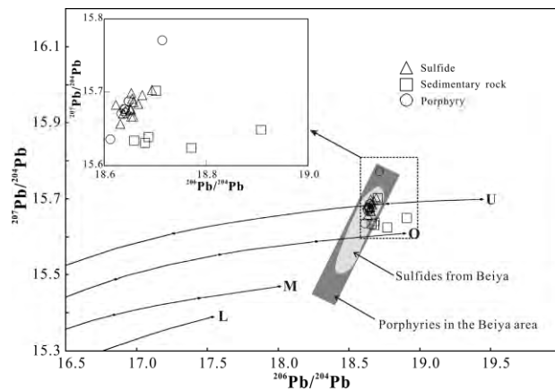
图 4 炉坪与北衙 Pb 同位素组成
