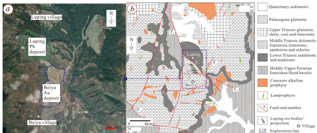
图 1 炉坪与北衙的空间关系 (a) 和区域地质简图 (b)
