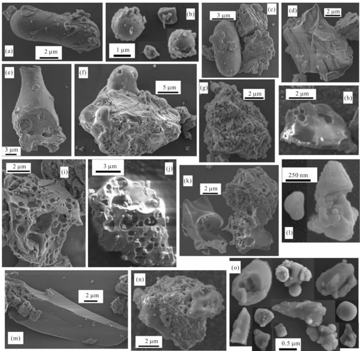
图 2 月尘颗粒基本形态的 SEM 图像,除了 j 图显示颗粒以外的所有颗粒均经过表面活性剂清洗处理(Liu et al. , 2006)
