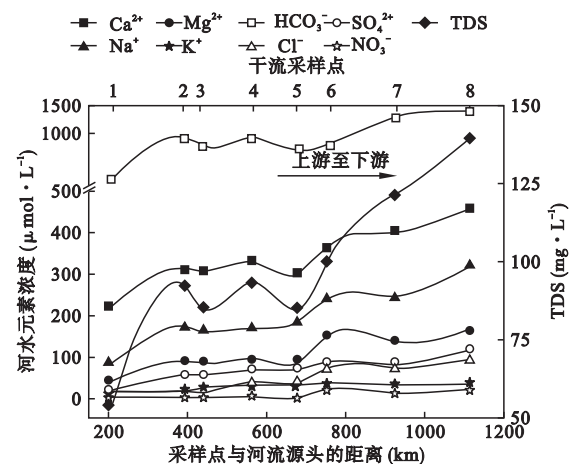
图 4 嫩江干流河水中各离子含量和 TDS 的沿程变化 Fig. 4 Variation of the ions and TDS in the Nenjiang main streams
