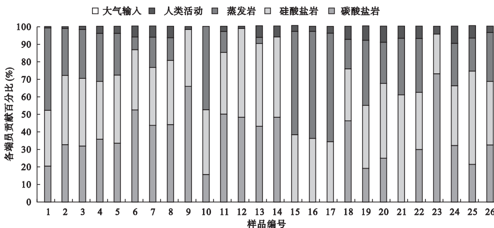
图 9 各端员对嫩江河水阳离子总量的贡献百分比
