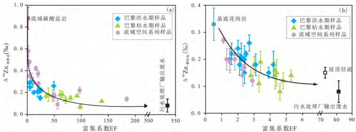
图1 塞纳河流域样品溶解态 \delta^{66}\text{Zn} 与富集系数的关系(a)以及颗粒态 \delta^{66}\text{Zn} 与富集系数的关系(b)
