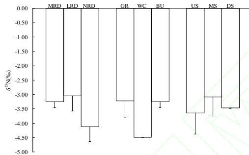
图 4 不同环境条件下黑色石灰土区地表凋落物 \delta^{15}\text{N} 均值
