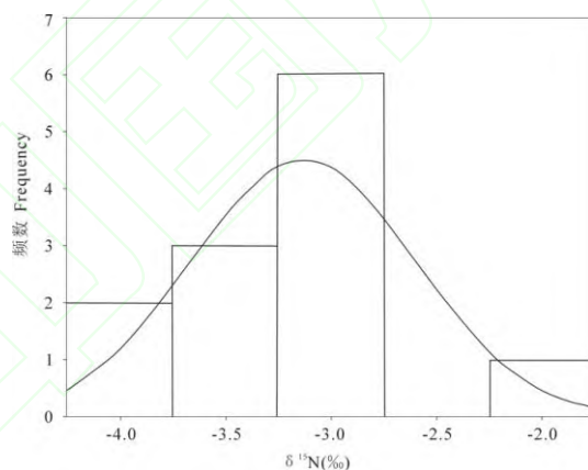
图1 黄壤区地表凋落物 \delta^{15}\text{N} 值的频数分布直方图
