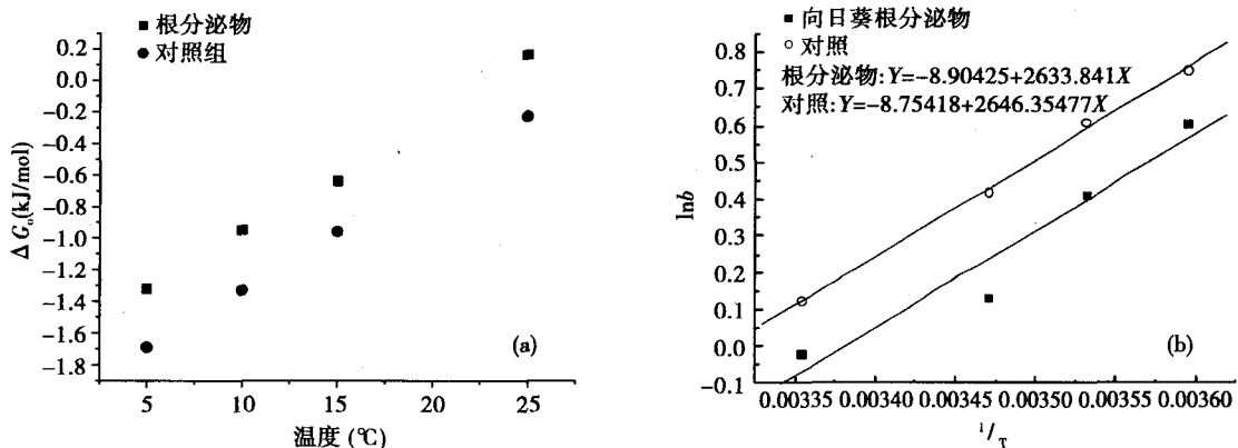
图 4 (a) 不同温度下针铁矿吸附 Cd 2+ 的自由能；(b) ln b 与 1/T 的线性关系
