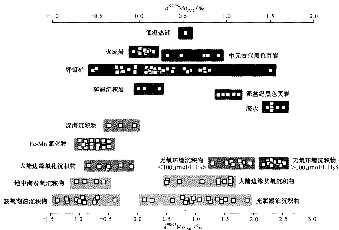
图 1 自然界中 Mo 同位素组成变化图 [数据引自 Siebert 等 (2003)、Barling 和 Anbar (2004)、Anbar 和 Rouxel (2007)、Malinovsky 等 (2007a, 2007b)]
