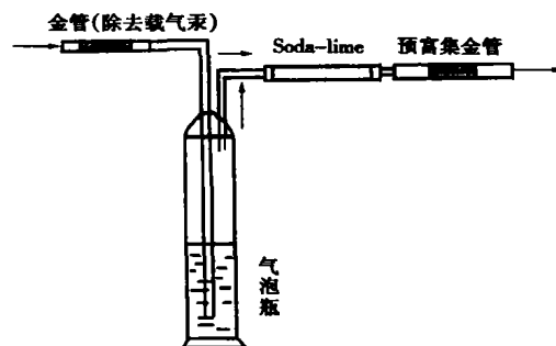
图 1 水样中汞的预富集原理
