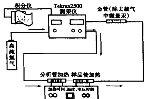
图 2 汞的仪器分析测定原理
