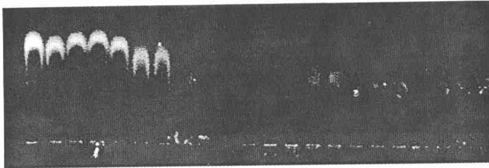
图3 洱海沉积物中DNA的紫外图像
