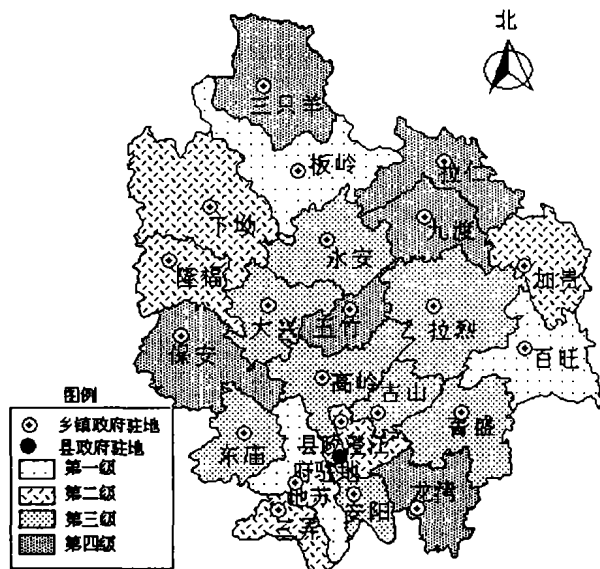
图 3 基于模型分析的都安县喀斯特石漠化的驱动力综合指数示意图
