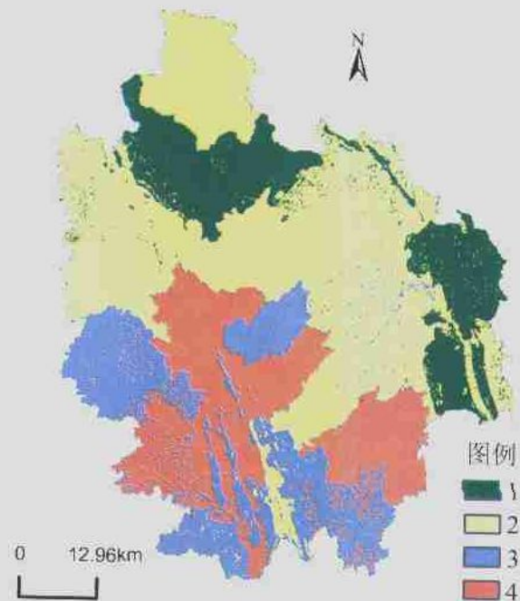
图 2 基于图谱分析的都安县喀斯特石漠化的驱动力综合指数分级图
